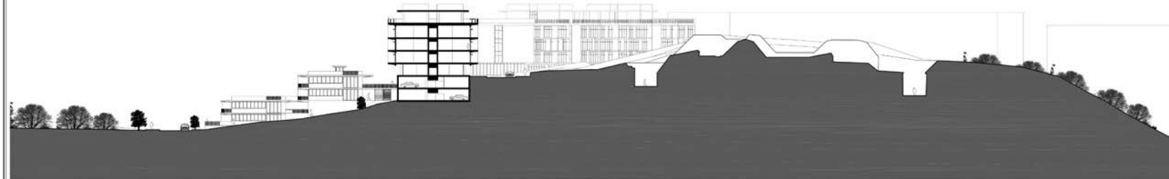
LONGITUDINAL SECTION B - B
